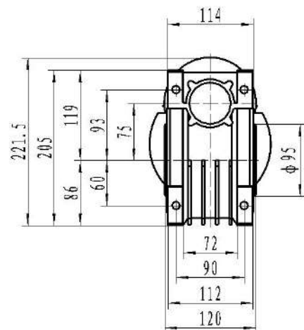
Ausgangshohlwelle / Output shaft hole
