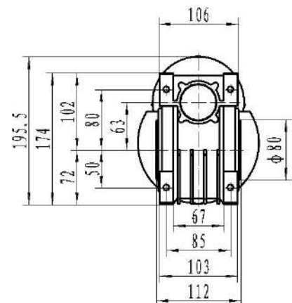
Ausgangshohlwelle / Output shaft hole
