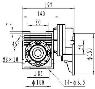
Eingangshohlwelle / Input shaft hole
