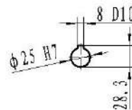
Ausgangshohlwelle / Output shaft hole
