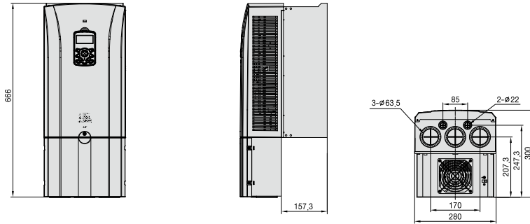
Drive + Conduit Box
