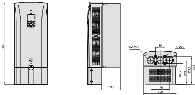
Drive + Conduit Box
