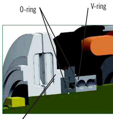
Labyrinthring aus Stahl- steel labyrinth ring
