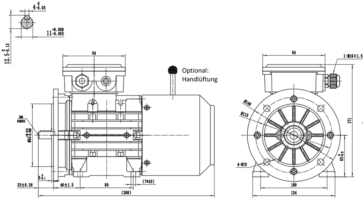
Typ / type SEV-BM3 632-2
