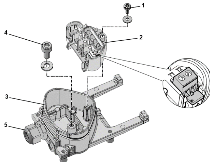
Fig. 24: Wiring
