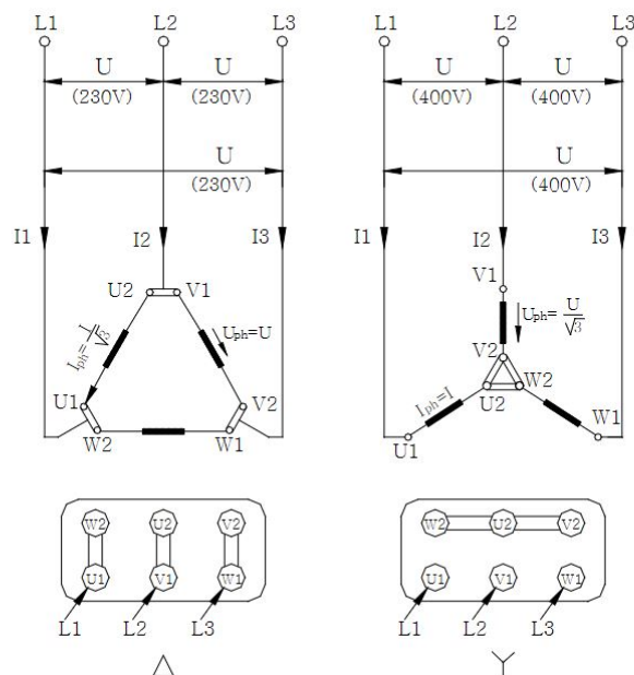
Elektrische Anschlussvarianten für den Getriebemotor
