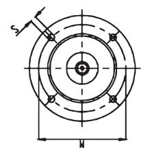
B5 Flansch / B5 Flange
